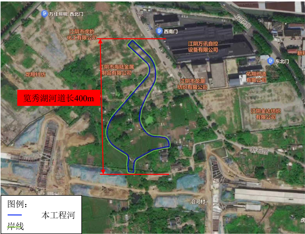
图2-7 本工程总平面布置图
